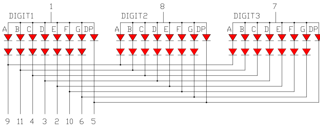
OPS-T8010LE-GW (Common Anode)
